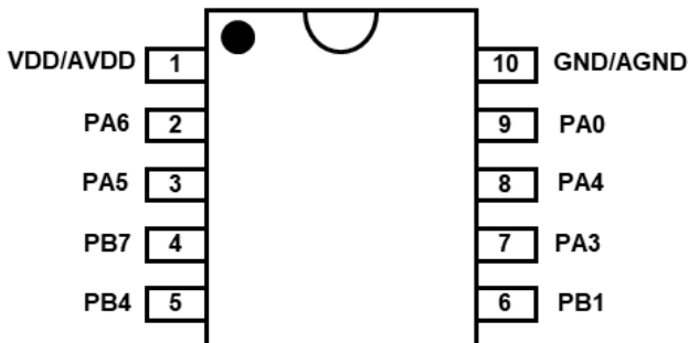
PFS122B-M10 (MSOP10-118mil)
